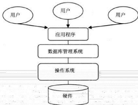
图 1.2 数据库系统
